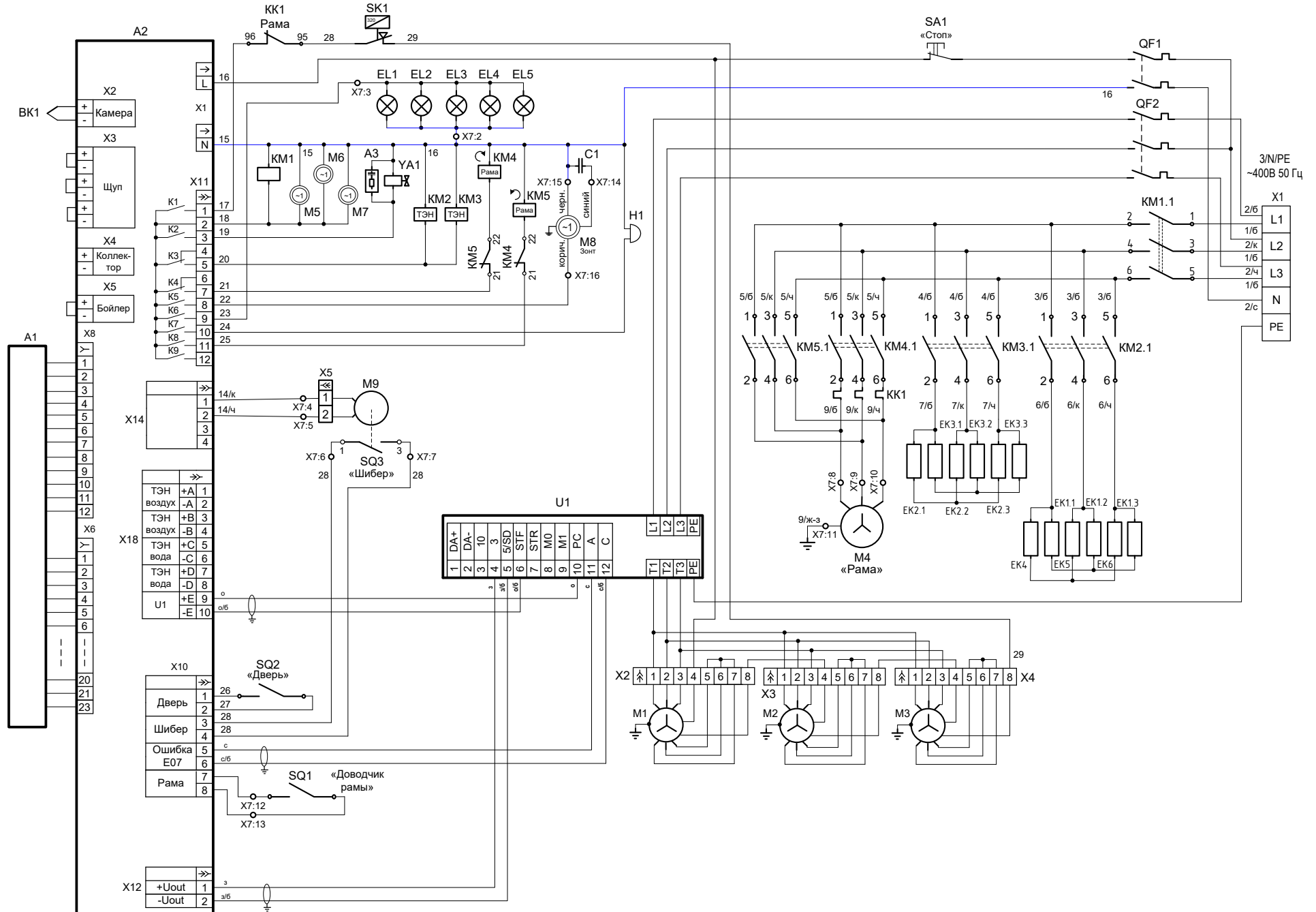
Рис. 9 - СХЕМА ЭЛЕКТРИЧЕСКАЯ ПРИНЦИПАЛЬНАЯ РПШ-18-8-6МР, РПШ-18-8-6ШР
