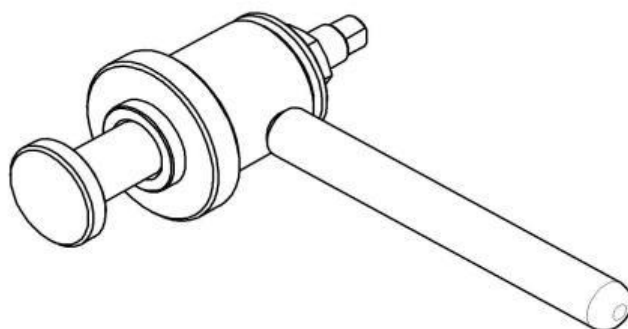
Рис. 10. Приспособление для запрессовки манжет(11000001333).
